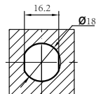
Otwór montażowy w metalu
