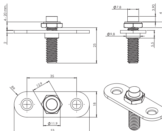
Zawias dolny
